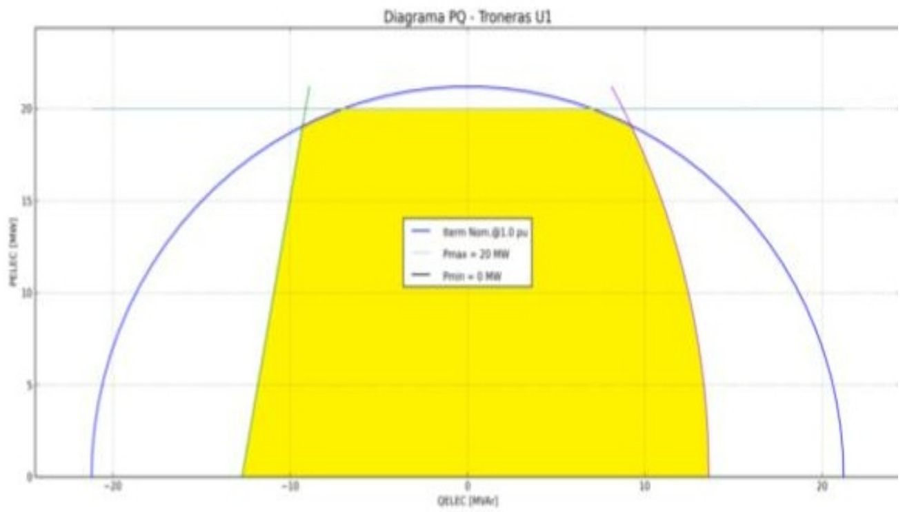
Figura 2: Curva de referencia probada y auditada unidad 1 Central Troneras según acuerdo CNO 1586 en el año 2025.
