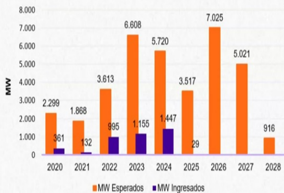
Capacidad esperada vs. Capacidad Ingresada anual
