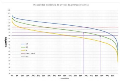
Generación térmica Verano 2015 -2016
