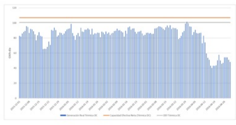
Generación térmica Verano 2015 -2016
