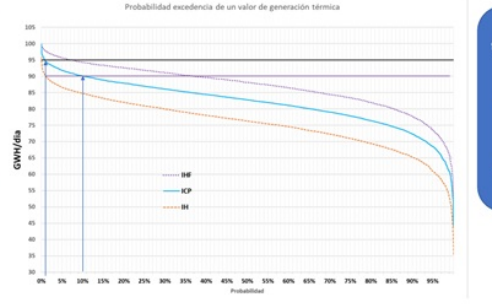
Distribución acumulada de las generación térmica Verano 2015 - 2016
