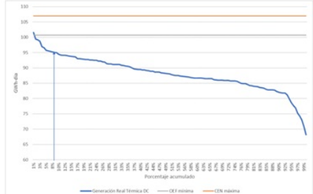
Distribución acumulada de las generación térmica Verano 2015 - 2016
